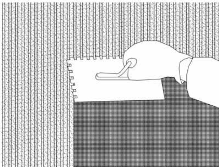
Влаштування армувального шару
