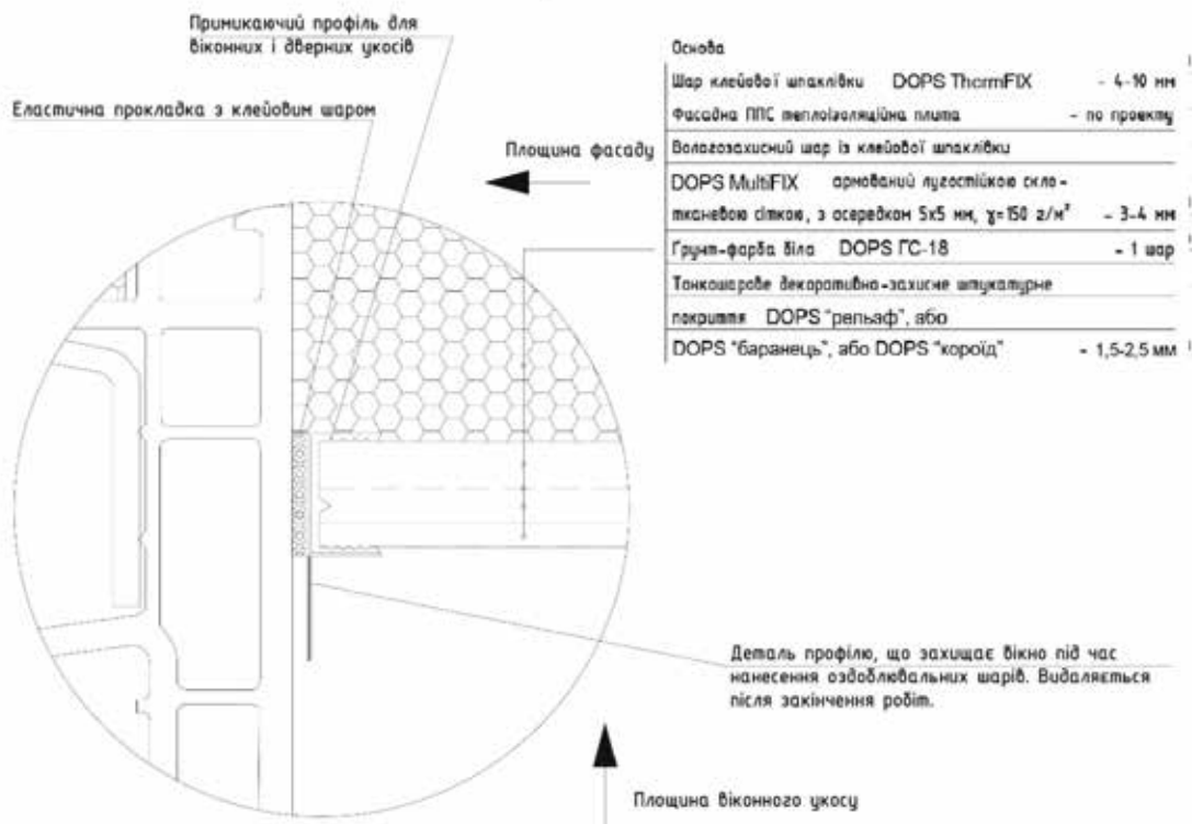
Вузол А.3.
