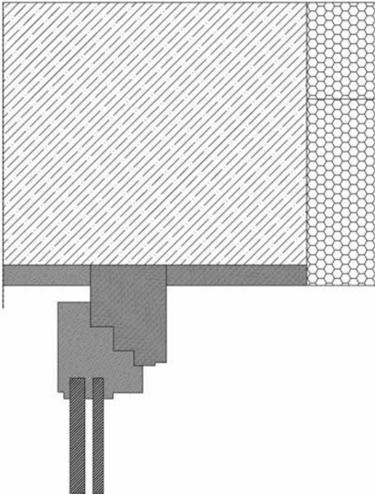
Влаштування армувального шару
